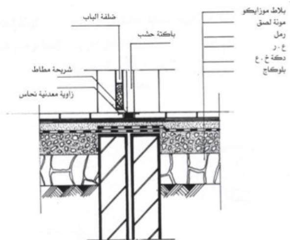
فواصل هيوط تمدد في أرضية مستمرة في الدور الأرضي
